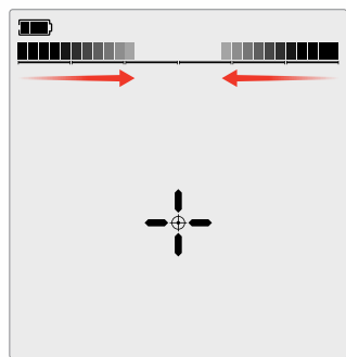
弱/偏离中心的目标信号：更少的判别区分段打开。目标位于更靠近探盘外侧的位置。
